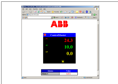
Fig. 3.1 Webservice
